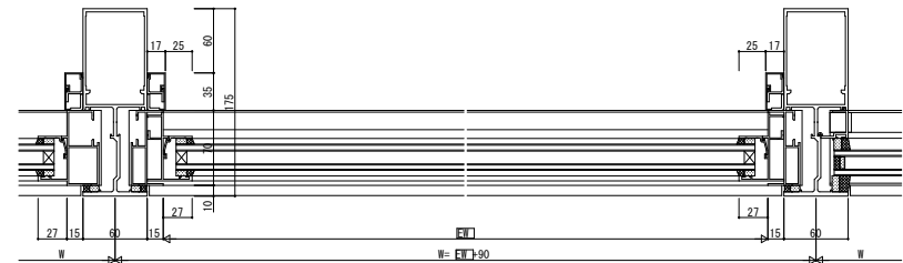
●FIX窓【内押縁タイプ】
