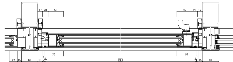
●たてすべり出し窓
