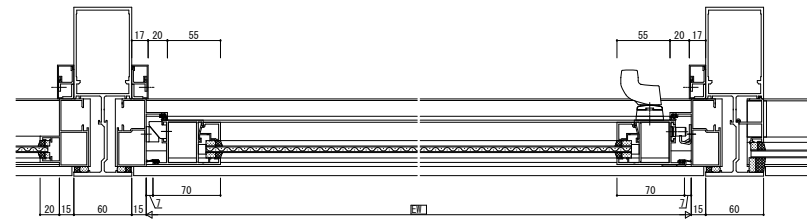
●たてすべり出し窓
