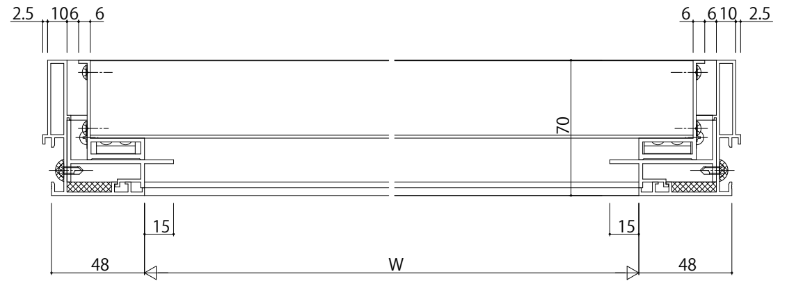
振れ止め部
