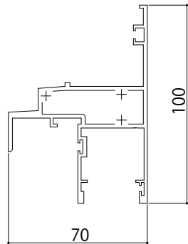
■外倒し・突出し【排煙窓・隠ぺい】／片引き [2K-84424]
