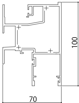
■FIX(18・28mm)／片引き [2K-84423]
