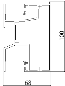
■FIX／FIX(18・28mm) [2K-95830]
