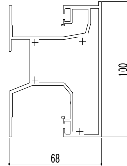
■FIX /FIX (18・38mm) [2K-84484]
