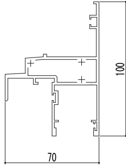
■外倒し・突出し【排煙窓・隠ぺい】 /片引き ■片引き /FIX (18・28mm) [2K-84424] [2K-84463]
