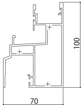
■片引き／FIX(18・28mm) [2K-84463]
