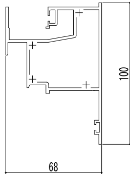
■外倒し・突出し【排煙窓・隠ぺい】 /FIX (38■)FIX (18・28mm) /可動 [2K-84487] [2K-95831]
