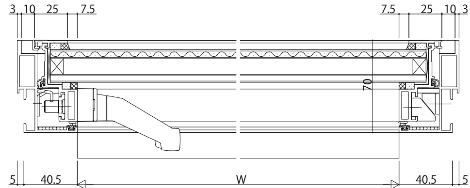
網戸受け用無目カバー
