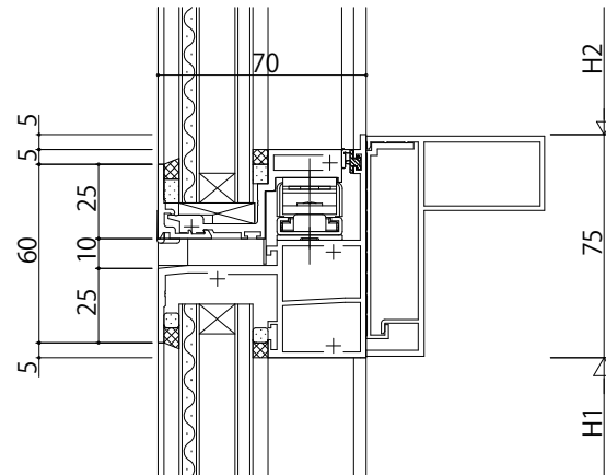
網戸受け用無目カバー
