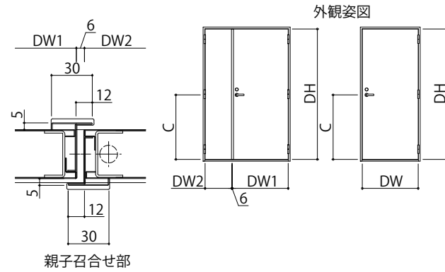
外観姿図
