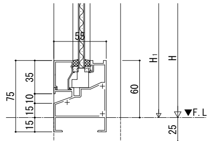
幅木75見付
