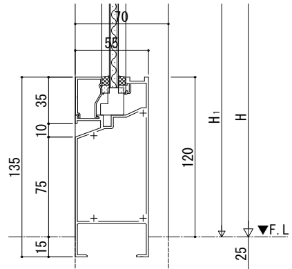
幅木135見付
