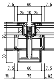
●可動窓/可動窓
