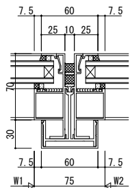
●FIX窓/FIX窓
