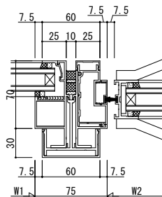
●FIX窓/フロアヒンジドア
