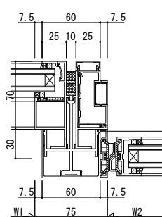
●FIX窓/自動ドア [片引き(戸先)]
