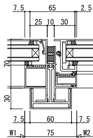
●FIX窓/片開きドア
