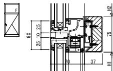
●FIX窓/たてすべり出し窓
