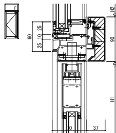
●外倒し窓（隠ぺい）/自由開きドア
