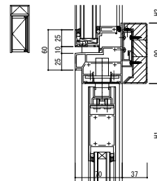
●突出し窓（隠ぺい）/自由開きドア
