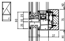
●たてすべり出し窓/FIX窓
