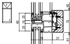
●外倒し窓（隠ぺい）/FIX窓
