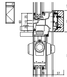
●FIX窓/片開きドア
