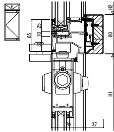
●外倒し窓（隠ぺい）/片開きドア
