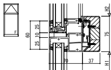
●突出し窓（隠ぺい）/FIX窓
