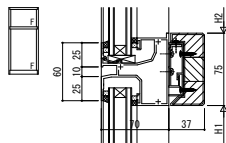
●FIX窓/FIX窓
