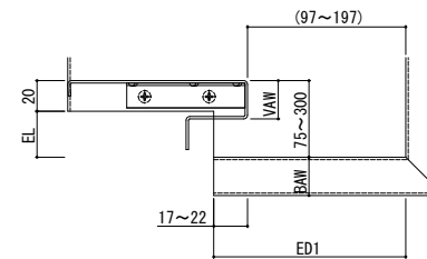
A-A部見上げ図
