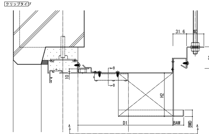
B矢視図
