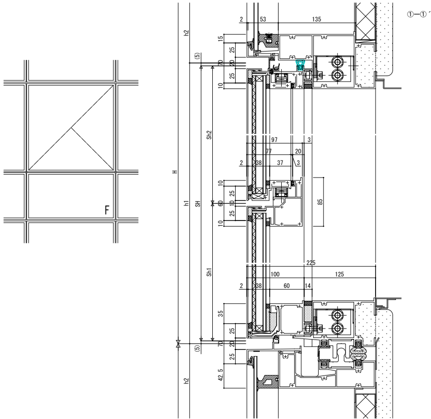
たてすべり出し窓/FIX窓 防火 換気仕様
