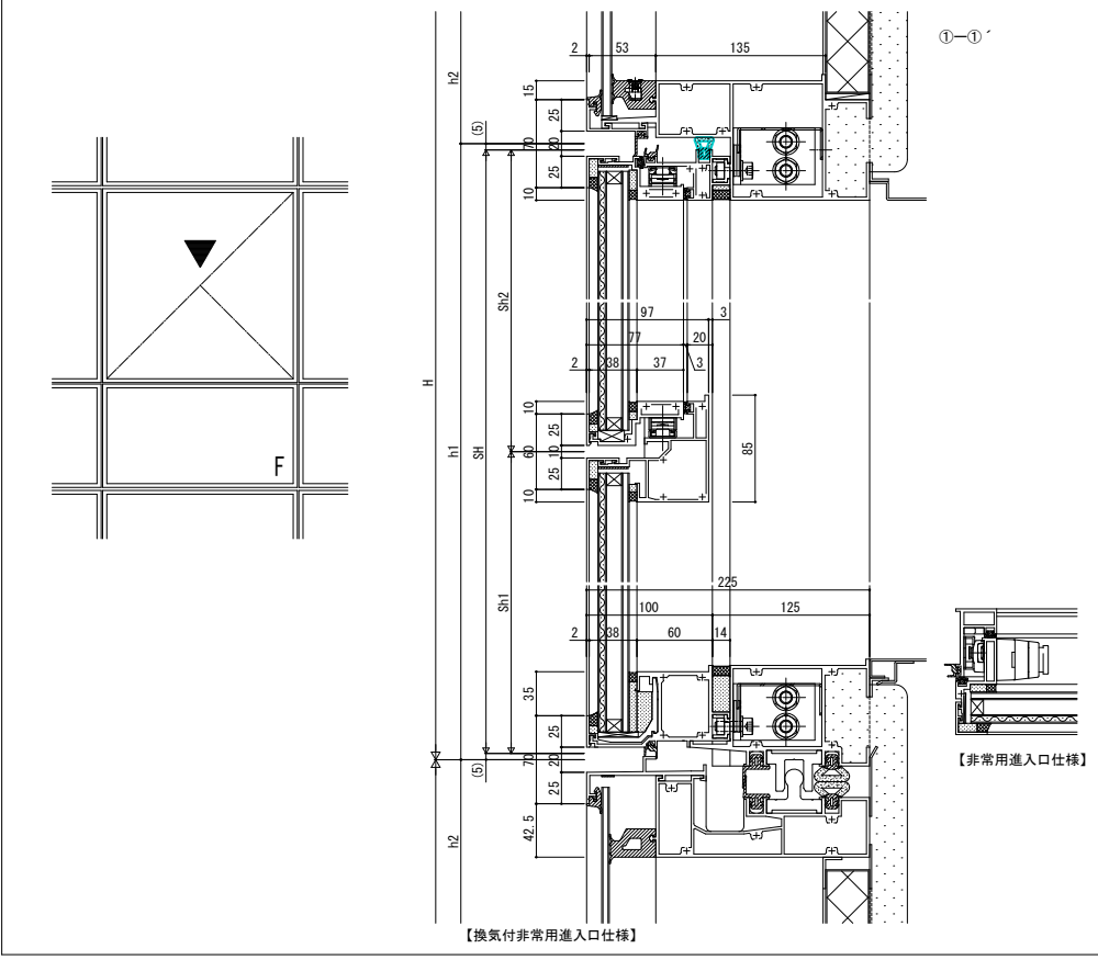
たてすべり出し窓/FIX窓 防火 非常用進入口仕様、換気付非常用進入口仕様
