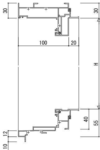
(9) たてすべり出し窓・突出し窓
