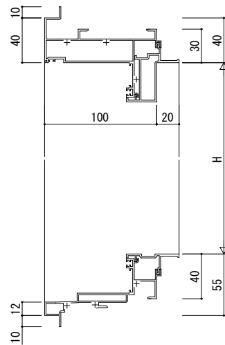
(8) たてすべり出し窓・突出し窓
