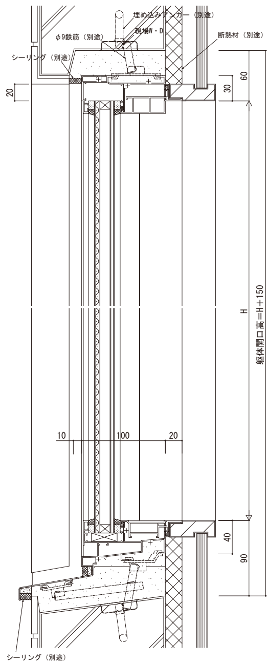
FIX窓
