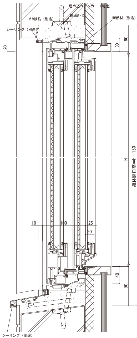
引違い窓
