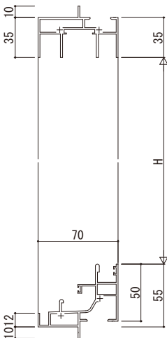
(3) 引違い窓・片引き窓 つらいち枠 アンゲルなし
