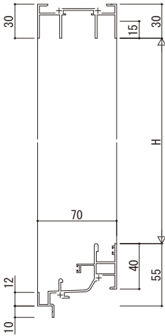
(2) 引違い窓・片引き窓 ALC枠 アンゲルなし
