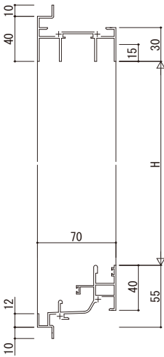
(2) 引違い窓・片引き窓 ALC枠 アンゲルなし
