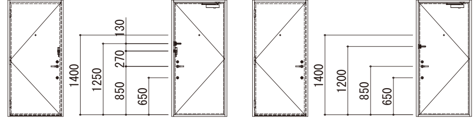
外観姿図
