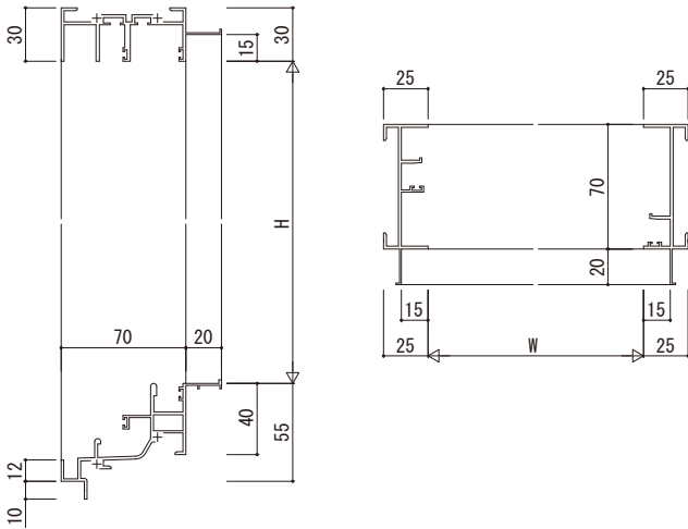
(3) 引違い窓・片引き窓・両袖片引き窓・引分け窓
