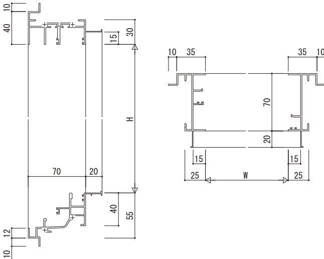
(3) 引違い窓・片引き窓・両袖片引き窓・引分け窓
