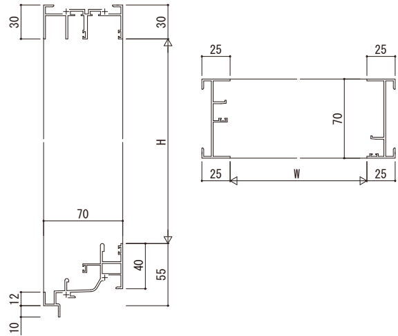
(4) 引違い窓・片引き窓・両袖片引き窓・引分け窓
