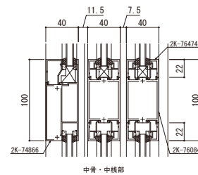
中骨・中横部
