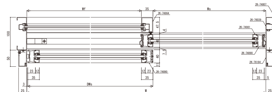
防護スクリーン付自動ドア
