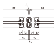
引分け突合せ部
