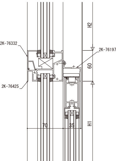
FIX窓／引込み戸
