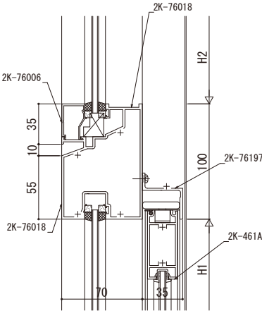
FIX窓／引込み戸
