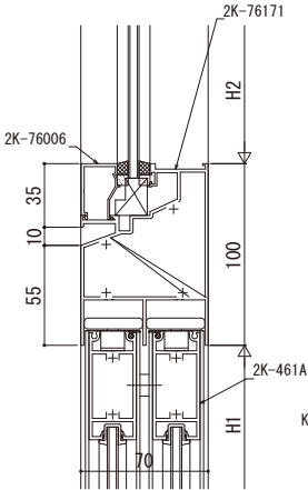
FIX窓／引違い戸
