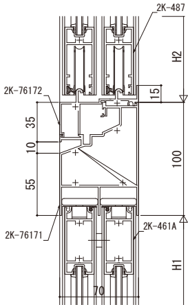
引違い窓／引違い戸
