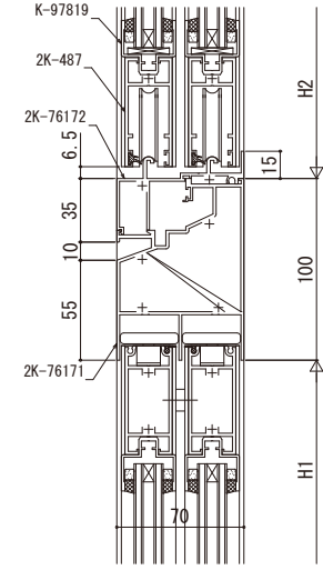
引違い窓／引違い戸
