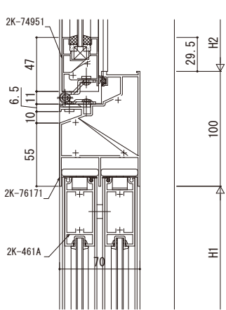
外倒し窓／引違い戸
