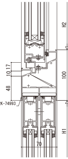
外倒し窓／引違い戸
