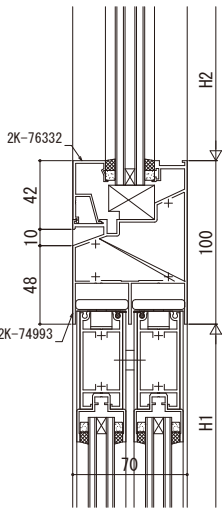
FIX窓／引違い戸
