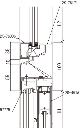
FIX窓／片引き戸・引分け戸
