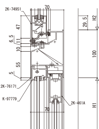
外倒し窓／片引き戸・引分け戸
