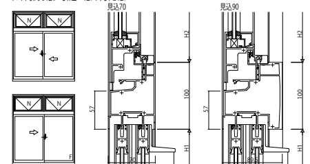
(8) 内倒し窓 / 引違い窓・片引き窓
