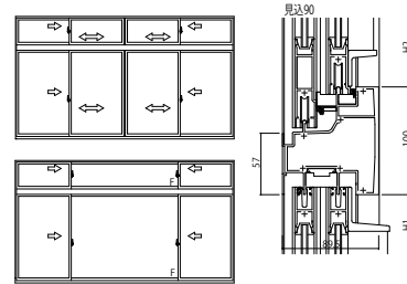
(3) 引違い窓(4枚建)・両袖片引き窓 / 引違い窓(4枚建)・両袖片引き窓
