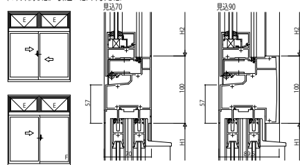
(6) 外倒し窓 / 引違い窓・片引き窓
