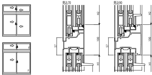
(1) 引違い窓・片引き窓 / 引違い窓・片引き窓
