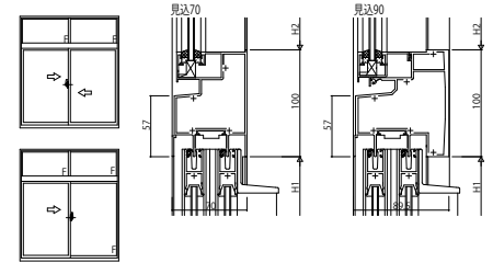
(4) F I X窓 / 引違い窓・片引き窓
