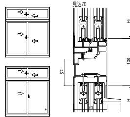
(2) 引違い窓(内外障子内はずし) / 引違い窓・片引き窓
