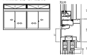
(7) 外倒し窓 / 引違い窓(4枚建)など
