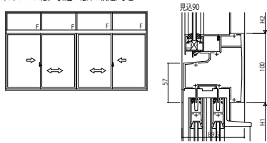
(5) F I X窓 / 引違い窓(4枚建)など
