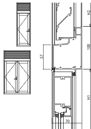
(78) 固定がらり(非脱着)ノドア(かまちタイプ)
