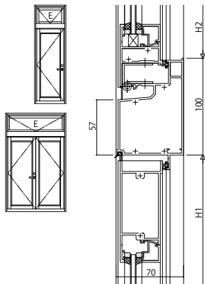
(77) 突出し窓(露出)ノドア(フラッシュタイプ)
