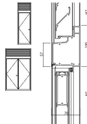
(79) 固定がらり(非脱着)ノドア(フラッシュタイプ)
