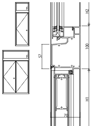
(75) 内倒し窓(露出・隠ぺい)ノドア(フラッシュタイプ)
