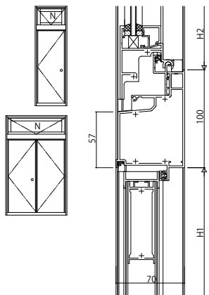
(80) 内開き窓・たて軸回転窓/FIX窓(内押縁) 60見付
