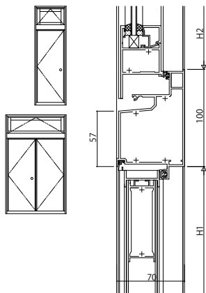
(77) 突出し窓(露出)ノドア(フラッシュタイプ)
