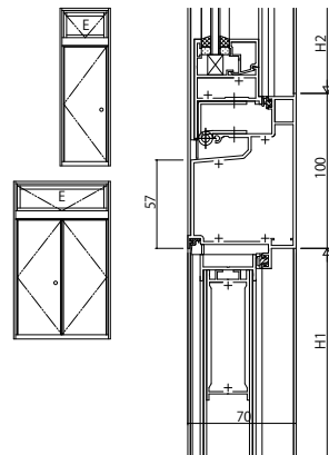
(78) 固定がらり(非脱着)ノドア(かまちタイプ)
