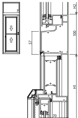
(76) 突出し窓(露出)ノドア(かまちタイプ)
