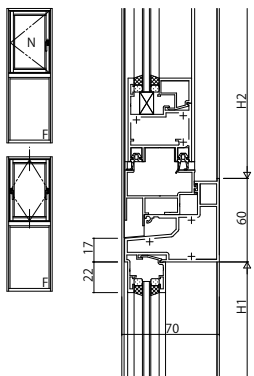
(80) 内開き窓・たて軸回転窓/FIX窓(内押縁) 60見付
