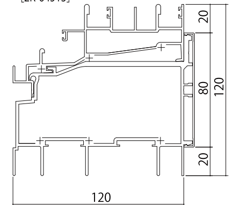
■引違い(3枚建)／(3枚建) [2K-64513]
