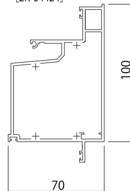
■FIX・可動／ドア [2K-64424]
