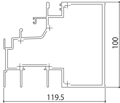
■引違い(4枚建)／引違い(4枚建) [2K-64517]
