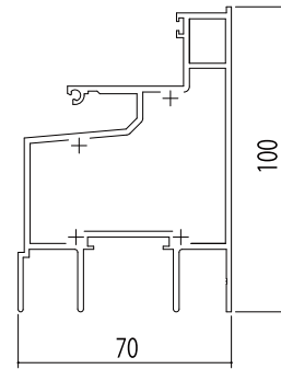
■外倒し・突出し／引違い・片引き [2K-64413]
