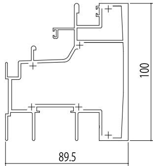
■引違い(4枚建)・両袖片引き／引違い(4枚建)・両袖片引き [2K-64471]
