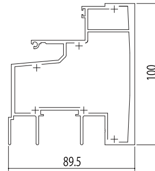
■FIX(内押縁)／引違い(4枚建)・両袖片引き [2K-64484]
