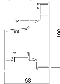
■可動/たて軸・内開き、FIX・たて軸(内開き) [2K-64505]
