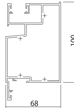
■可動/たて軸・内開き、FIX・たて軸(内開き) [2K-64505]
