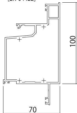
■FIX／可動※ 可動／可動※ [2K-64422]
