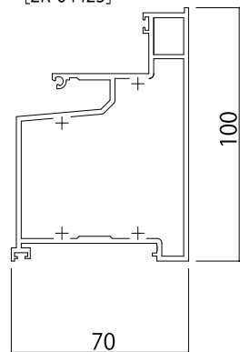
■FIX／内倒し 内倒し／内倒し [2K-64423]
