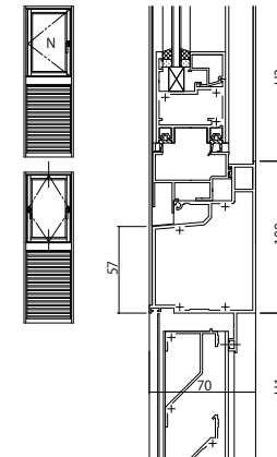
(88) 引違い窓(4枚建)・両袖片引き窓/引違い窓(4枚建)・両袖片引き窓
