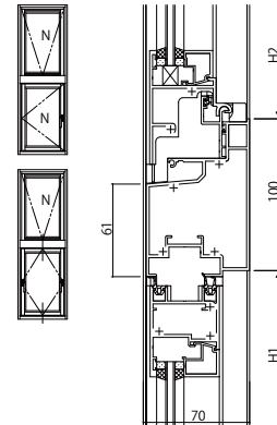
(83) 内倒し窓(一般・露出・隠べい)/内開き窓・たて軸回転窓
