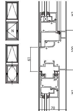
(84) 突き出し窓(カムラッチ・露出)/内開き窓・たて軸回転窓
