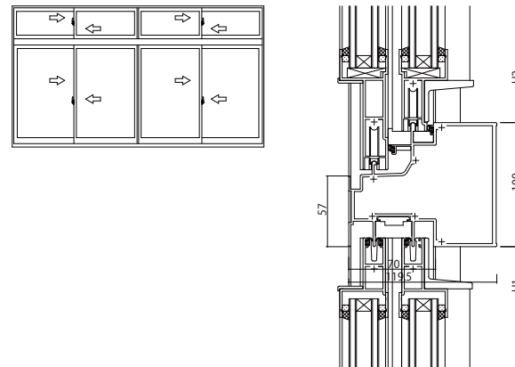
(88) 引違い窓(4枚建)・両袖片引き窓/引違い窓(4枚建)・両袖片引き窓
