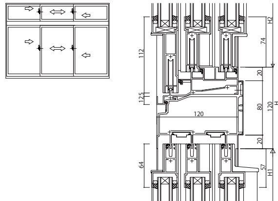
(87) 引違い窓(3枚建)/引違い窓(3枚建)
