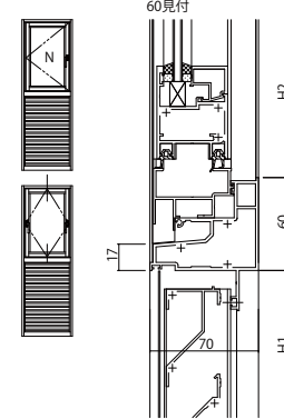
(86) 内開き窓・たて軸回転窓/固定がらり(非脱着)
