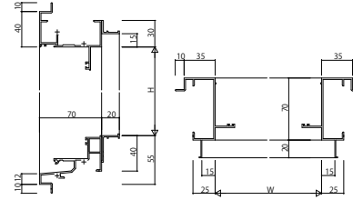
(19) 可動窓 ※1※3 設備枠 (内付) アングルなし
