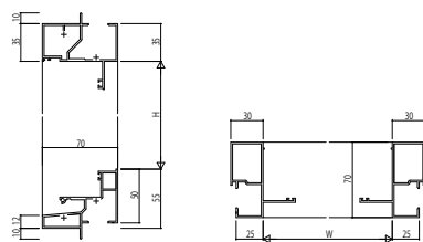
(22) 外側し窓【開けいオペレーター】・突出し窓【開けいオペレーター】・たてすべり出し窓【オペレーターハンドル】(スリット換気) ついで枠 アングルなし
