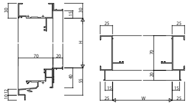
(17) 可動窓 ※1※3 ついで枠 アングルなし
