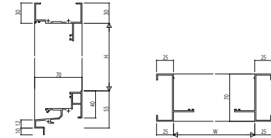
(24) 内側し窓 ※2 RC枠 アングルなし
