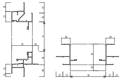
(18) 可動窓 ※1※3 設備枠 (半外付) アングルなし
