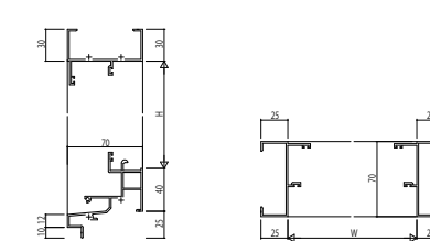
(24) 内側し窓 ※2 RC枠 アングルなし
