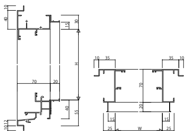
(25) 内側し窓 ※2 ALC枠 アングル付
