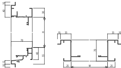
(21) 外側し窓【開けいオペレーター】・突出し窓【開けいオペレーター】・たてすべり出し窓【オペレーターハンドル】(スリット換気) ALC枠 アングルなし
