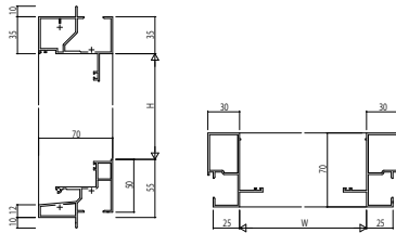
(17) 可動窓 ※1※3 ついで枠 アングルなし
