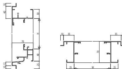
(26) 内側し窓 ※2 ALC枠 アングルなし
