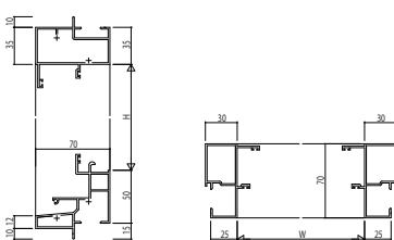
(27) 内側し窓 ※2 ついで枠 アングルなし
