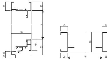
(18) 可動窓 ※1※3 設備枠 (半外付) アングルなし
