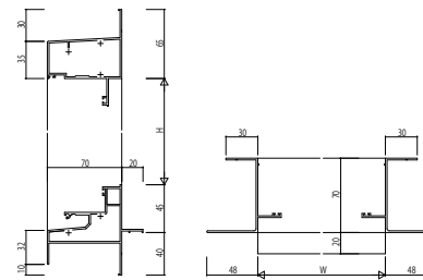
(19) 可動窓 ※1※3 設備枠 (内付) アングルなし
