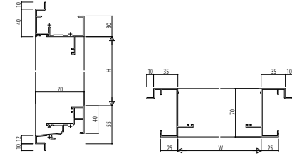
(20) 外側し窓【開けいオペレーター】・突出し窓【開けいオペレーター】・たてすべり出し窓【オペレーターハンドル】(スリット換気) RC枠 アングルなし
