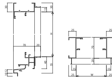
(23) 内側し窓 ※2 RC枠 アングル付
