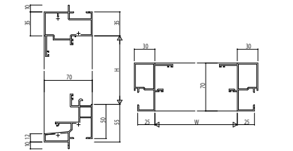
(37)内側窓【排煙窓・露出オペレーター仕様】 つらいち枠 アングルなし
