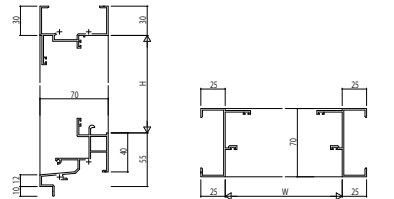
(35)内側窓【排煙窓・露出オペレーター仕様】 RC枠 アングルなし
