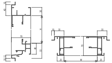
(31)内側窓【排煙窓・排煙鏡】・内側窓【排煙窓・露出オペレーター仕様】 ALC枠 アングルなし
