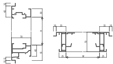
(39)内開き ALC枠 アングルなし
