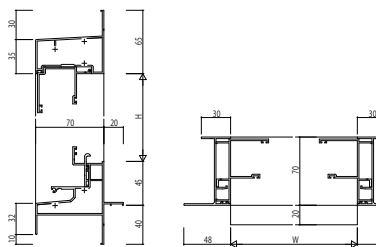
(34)内側窓【排煙窓・排煙鏡】・内側窓【排煙窓・露出オペレーター仕様】 鉄骨枠(引引) アングルなし
