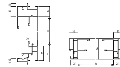
(32)内側窓【排煙窓・排煙鏡】・内側窓【排煙窓・露出オペレーター仕様】 つらいち枠 アングルなし
