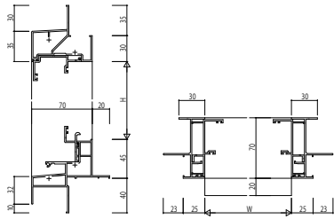
(28)内側窓 #2 鉄骨枠 (半外付)アングルなし
