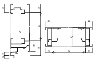
(38)内開き RC枠 アングルなし
