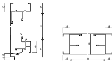
(34)内側窓【排煙窓・排煙鏡】・内側窓【排煙窓・露出オペレーター仕様】 鉄骨枠(引引) アングルなし
