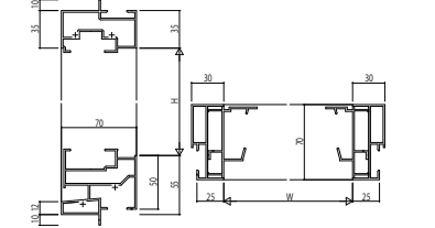
(40)内開き つらいち枠 アングルなし
