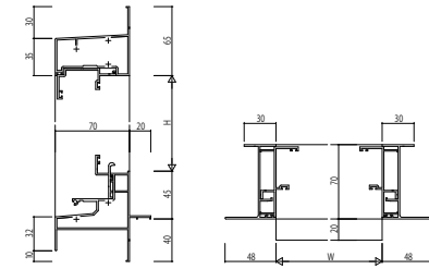
(29)内側窓 #2 鉄骨枠 (外付)アングルなし
