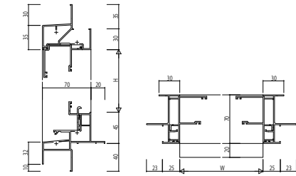
(33)内側窓【排煙窓・排煙鏡】・内側窓【排煙窓・露出オペレーター仕様】 鉄骨枠 (半外付)アングルなし
