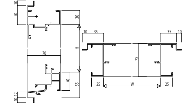
(36)内側窓【排煙窓・露出オペレーター仕様】 ALC枠 アングルなし
