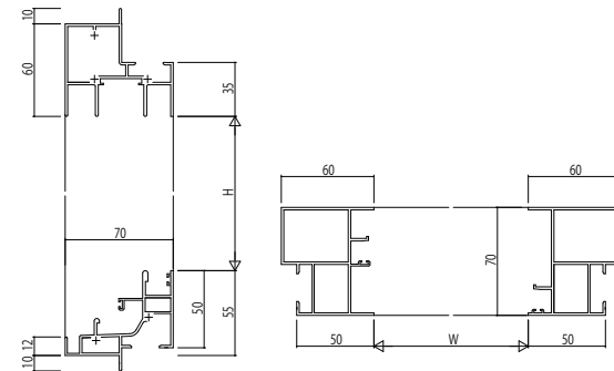
(6) 引違い窓・片引き窓・両袖片引き窓・引分け窓・自由片引き窓 自立(ついで枠) アンクルなし
