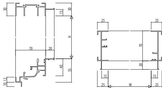
(1) 引違い窓・片引き窓・両袖片引き窓・引分け窓・自由片引き窓 RC枠 アンクル付
