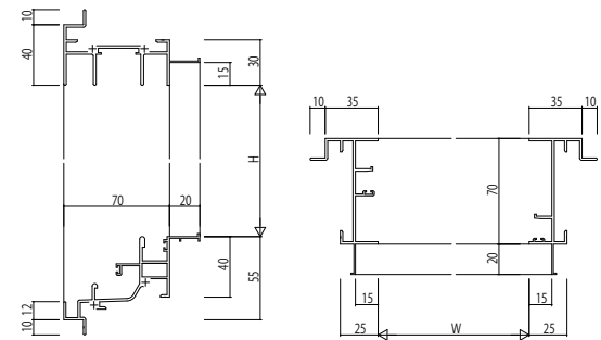
(3) 引違い窓・片引き窓・両袖片引き窓・引分け窓・自由片引き窓 ALC枠 アンクル付
