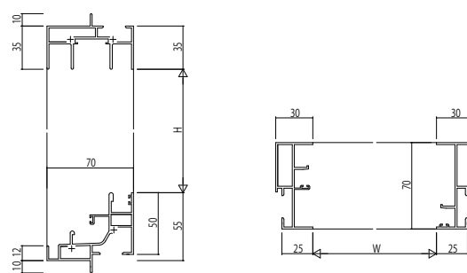
(5) 引違い窓・片引き窓・両袖片引き窓・引分け窓・自由片引き窓 ついで枠 アンクルなし
