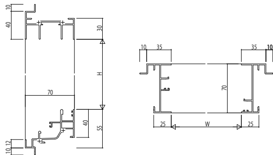
(4) 引違い窓・片引き窓・両袖片引き窓・引分け窓・自由片引き窓 ALC枠 アンクルなし
