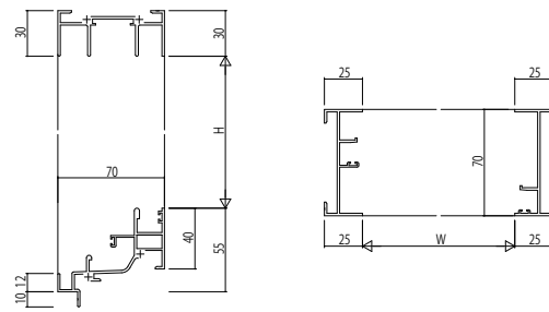
(2) 引違い窓・片引き窓・両袖片引き窓・引分け窓・自由片引き窓 RC枠 アンクルなし
