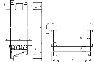
(12) 引違い窓・片引き窓(下枠フラット仕様) ALC枠 アングル付
