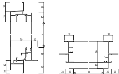
(7) 引違い窓・片引き窓・両軸片引き窓・引分け窓・自由片引き窓 鉄骨枠 単外付
