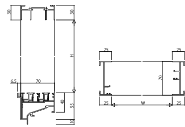
(11) 引違い窓・片引き窓(下枠フラット仕様) RC枠 アングルなし
