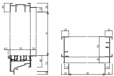
(10) 引違い窓・片引き窓(下枠フラット仕様) RC枠 アングル付
