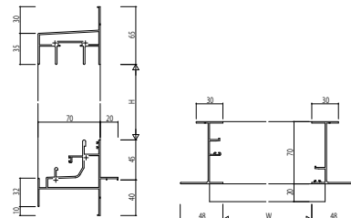
(8) 引違い窓・片引き窓・両軸片引き窓・引分け窓・自由片引き窓 鉄骨枠 外付
