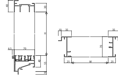
(13) 引違い窓・片引き窓(下枠フラット仕様) ALC枠 アングルなし
