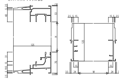
(9) 引違い窓 モッド/バック枠 アングルなし
