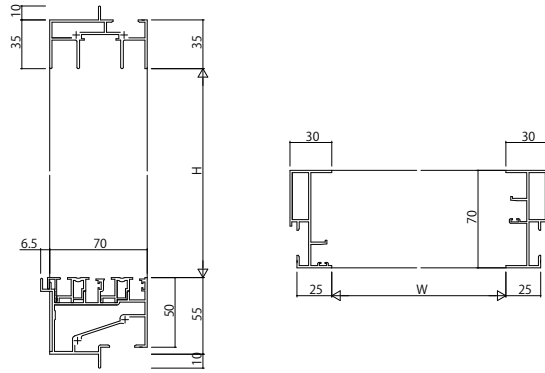
(17) 引違い窓・片引き窓(フラット下枠) 鉄骨枠 外付
