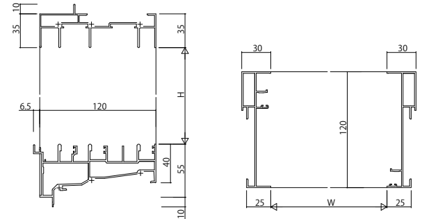
(21) 引違い窓(3枚建・6枚建)【レールフラット下枠】/【レールフラット下枠/緩衝ゴム付】 つらいち枠 アングルなし
