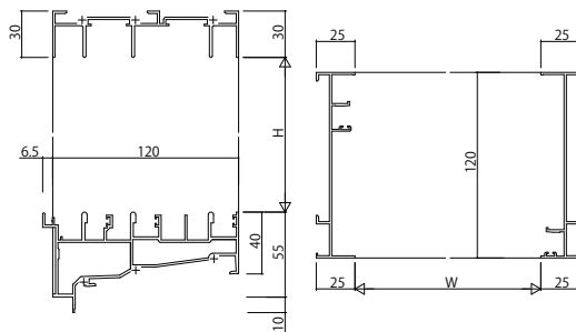
(20) 引違い窓(3枚建・6枚建)【レールフラット下枠】/【レールフラット下枠/緩衝ゴム付】 RC枠 アングルなし
