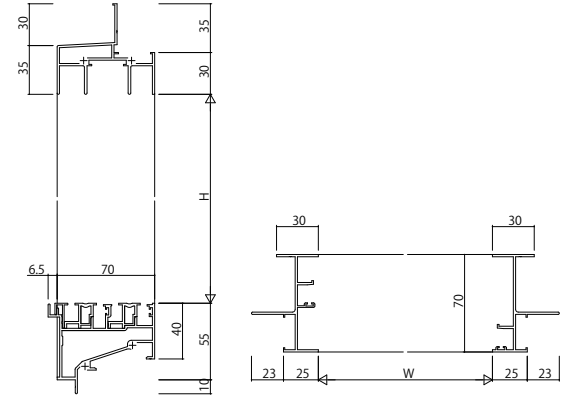
(16) 引違い窓・片引き窓(フラット下枠) 鉄骨枠 半外付
