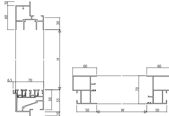
(18) 引違い窓【カウンター窓】 RC枠 アングルなし
