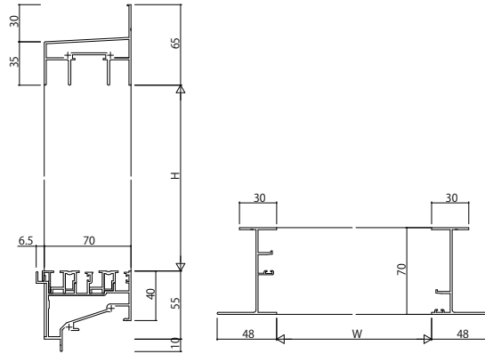
(17) 引違い窓・片引き窓(フラット下枠) 鉄骨枠 外付
