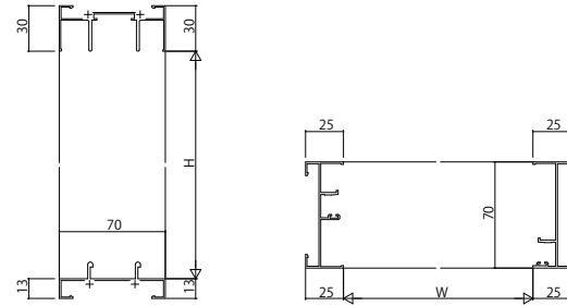
(18) 引違い窓【カウンター窓】 RC枠 アングルなし
