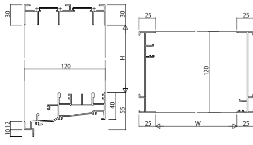
(19) 引違い窓(3枚建・6枚建)・引違い窓(3枚建・6枚建)【緩衝ゴム付】 RC枠 アングルなし
