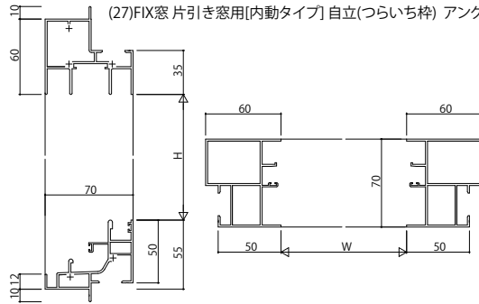
(27)FIX窓片引き窓用[内動タイプ] 自立(つらいち枠) アングルなし
