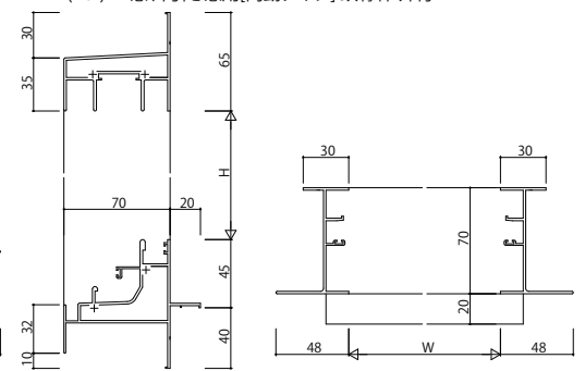
(29)FIX窓片引き窓用[内動タイプ] 鉄骨枠 外付
