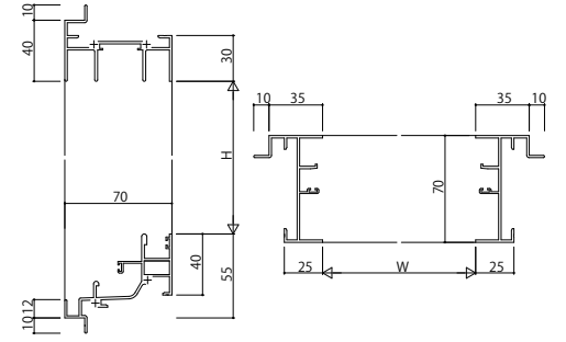
(25)FIX窓片引き窓用[内動タイプ] ALC 枠 アングルなし
