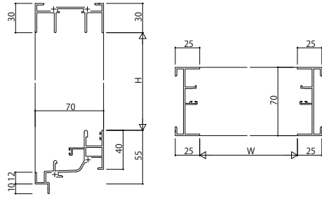
(23)FIX窓片引き窓用[内動タイプ] RC 枠 アングルなし
