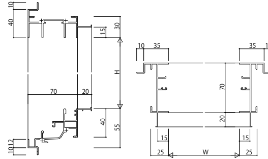
(24)FIX窓片引き窓用[内動タイプ] ALC 枠 アングル付
