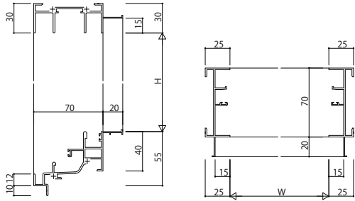
(22)FIX窓片引き窓用[内動タイプ] RC 枠 アングル付
