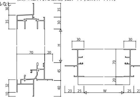
(28)FIX窓片引き窓用[内動タイプ] 鉄骨枠 半外付
