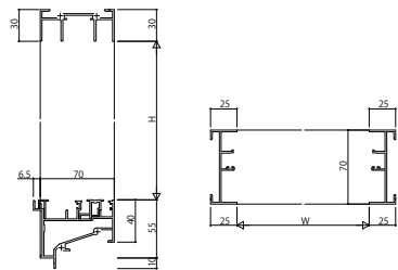
(31)FIX窓片引き窓用(内動・フラット下枠)RC種 アングルなし
