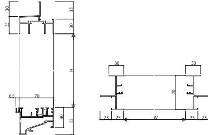
(36)FIX窓片引き窓用(内動・フラット下枠)鉄骨種 半外付
