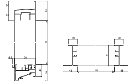
(37)FIX窓片引き窓用(内動・フラット下枠)鉄骨種 外付
