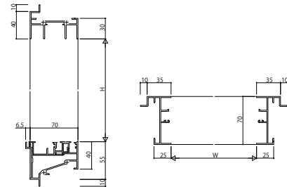
(33)FIX窓片引き窓用(内動・フラット下枠)ALC種 アングルなし
