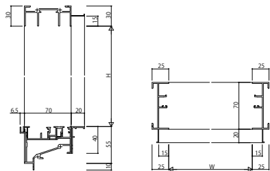
(30)FIX窓片引き窓用(内動・フラット下枠)RC種 アングル付
