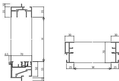
(34)FIX窓片引き窓用(内動・フラット下枠)つらいち種
