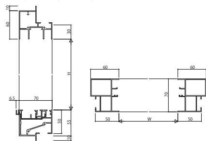
(35)FIX窓片引き窓用(内動・フラット下枠)自立(つらいち)種
