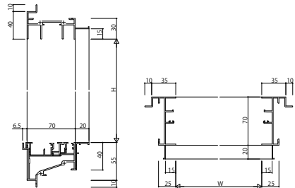
(32)FIX窓片引き窓用(内動・フラット下枠)ALC種 アングル付
