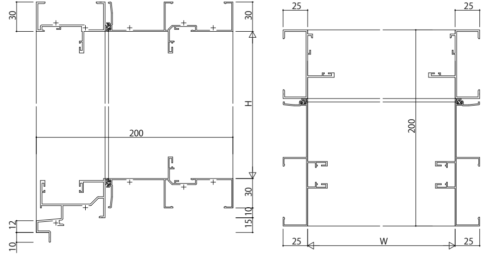
(52)二重窓【FIX窓】 RC枠 アングルなし
