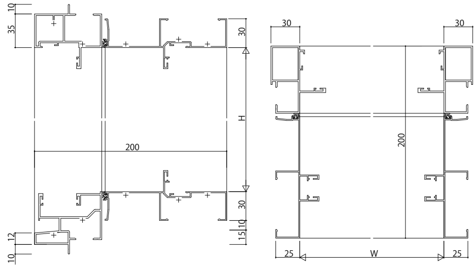
(54)二重窓【FIX窓】 つらいち枠 アングルなし
