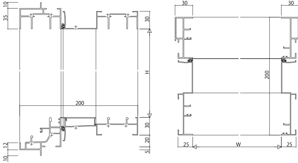
(51)二重窓【引違い窓】 つらいち枠 アングルなし
