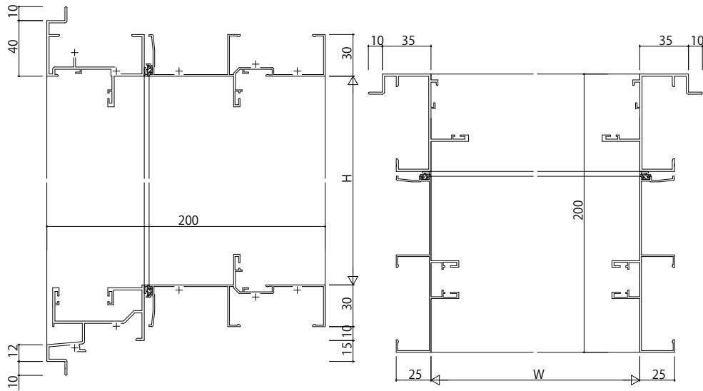
(53)二重窓【FIX窓】 ALC枠 アングルなし
