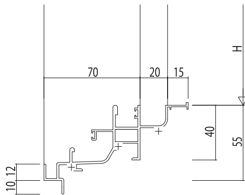
RC 枠 結露受一体枠 (55見付タイプ)
