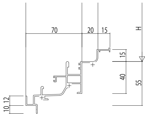
RC 枠 結露受一体枠 (70見付タイプ)
