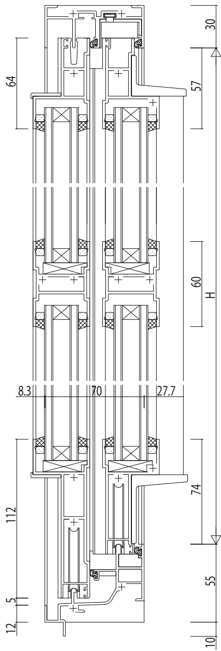
4枚建 Cタイプの場合
