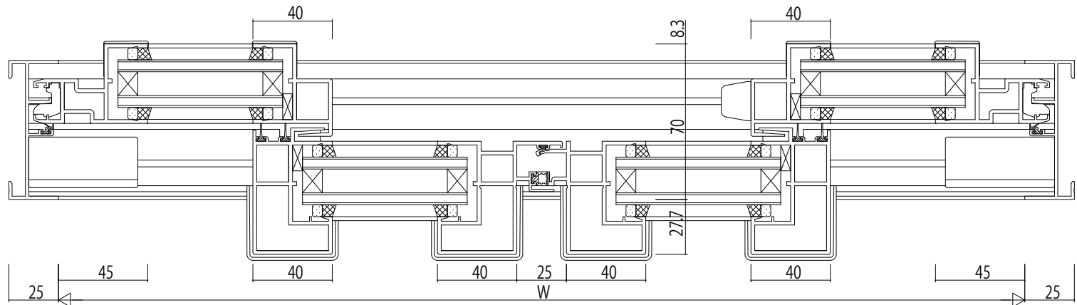
4枚建 Cタイプの場合
