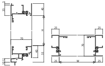
(9) FIX窓【内押線】 RC枠 アンガルなし
