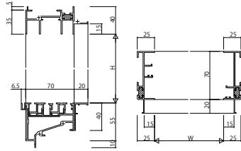
(3) 引違い窓・両袖片引き窓・引分け窓(フラット下枠) RC枠 アンガル付
