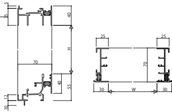
(10) 可動窓※1 RC枠 アンガルなし
