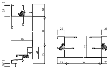
(13) 内倒し窓【排煙窓・排煙錠仕様】・ 内倒し窓【排煙窓・露出オペレーター仕様】 RC枠 アンガルなし
