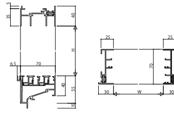
(12) 内倒し窓※2 RC枠 アンガルなし
