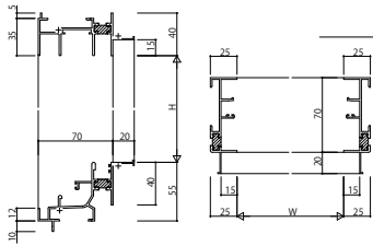
(9) FIX窓【内押線】 RC枠 アンガルなし
