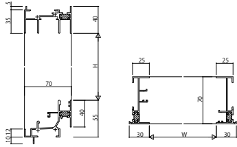
(2) 引違い窓・両袖片引き窓・引分け窓 RC枠 アンガルなし
