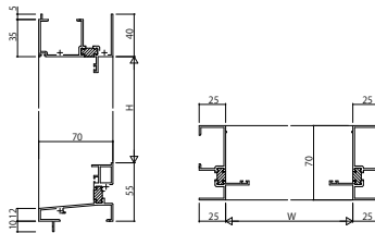
(14) 片開きドア / 両開きドア RC枠 アンガルなし
