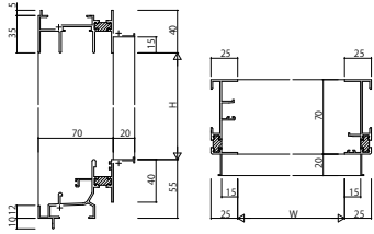
(1) 引違い窓・両袖片引き窓・引分け窓 RC枠 アンガル付
