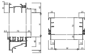
(11) 外倒し窓【排煙窓・隠ぺいオペレーター仕様】・ 突出し窓【排煙窓・隠ぺいオペレーター仕様】・ たてすべり出し窓【オペレーターハンドル仕様】【スリット換気仕様】 RC枠 アンガルなし
