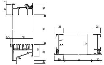
(4) 引違い窓・両袖片引き窓・引分け窓(フラット下枠) RC枠 アンガルなし
