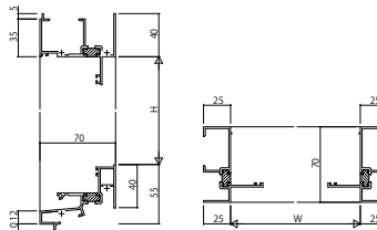
(11) 外倒し窓【排煙窓・隠ぺいオペレーター仕様】・ 突出し窓【排煙窓・隠ぺいオペレーター仕様】・ たてすべり出し窓【オペレーターハンドル仕様】【スリット換気仕様】 RC枠 アンガルなし
