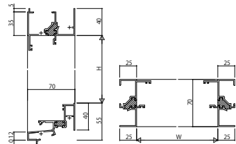
(12) 内倒し窓※2 RC枠 アンガルなし
