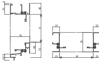
(10) 可動窓※1 RC枠 アンガルなし
