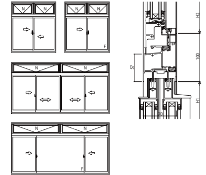
(4) 内倒し窓/引違い窓・片引き窓・両袖片引き窓・引違い窓(4枚建)
