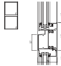
(7) FIX窓(内押縁)/FIX窓(内押縁)
