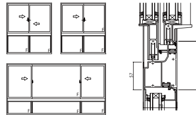
(6) 引違い窓・片引き窓・両袖片引き窓/FIX窓(内押縁)
