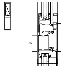
(12) たてすべり出し窓(オペレーターハンド/ル・スリット換気) / (13) FIX窓(内押縁)/外倒し窓(一般・露出) FIX窓(内押縁)
