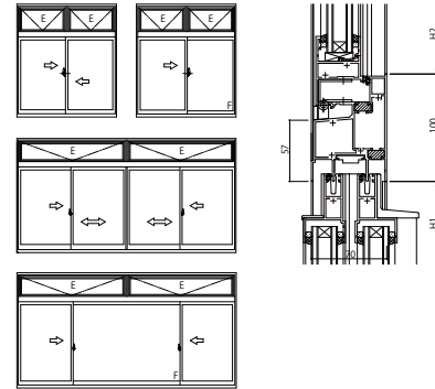
(3) 外倒し窓/引違い窓・片引き窓・両袖片引き窓・引違い窓(4枚建)
