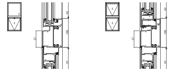
(12) たてすべり出し窓(オペレーターハンド/ル・スリット換気) / (13) FIX窓(内押縁)/外倒し窓(一般・露出) FIX窓(内押縁)
