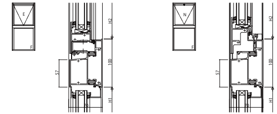
(8) 外倒し窓(一般・露出・隠べい)/FIX窓(内押縁) (9) 内倒し窓(一般・露出)/FIX窓(内押縁)
