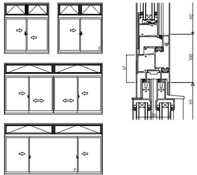
(5) 突出し窓/引違い窓・片引き窓・両袖片引き窓・引違い窓(4枚建)
