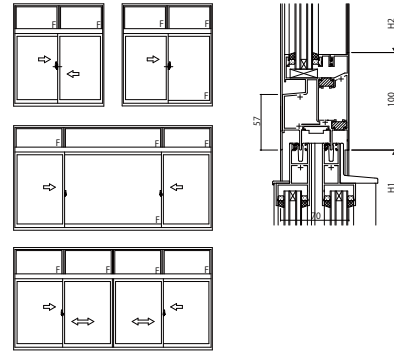
(2) FIX窓/引違い窓・片引き窓・両袖片引き窓・引違い窓(4枚建)
