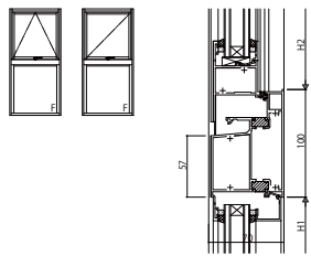
(10) 突出し窓(カムラッチ・露出)・すべり出し/FIX窓(内押縁)
