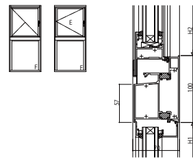
(11) 外開き窓・たてすべり出し窓/FIX窓(内押縁)
