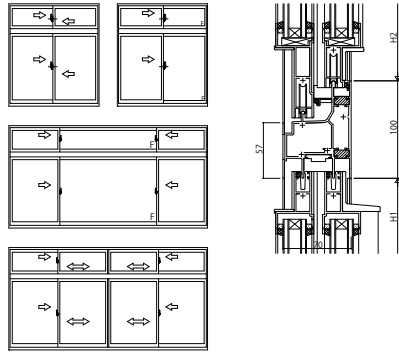
(1) 引違い窓・片引き窓・両袖片引き窓/引違い窓・片引き窓・両袖片引き窓 引違い窓(4枚建)/引違い窓(4枚建)
