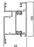
■FIX/FIX[2BK-61085]
