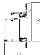
■可動/ドア[2BK-61092]
