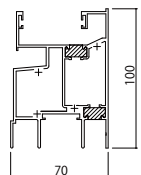
■FIX/引違い・片引き[2BK-61083]
