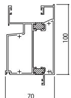
■FIX/ドア[2BK-61087]
