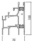
■引違い・片引き/ 引違い・片引き[2BK-61081]
