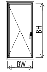
内観姿図(1:20)
