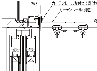
●カーテンレール対応ふかし枠25取付時
