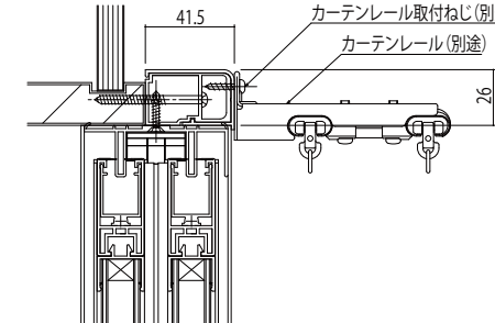
●カーテンレール対応ふかし枠40取付時
