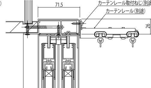
●カーテンレール対応ふかし枠70取付時
