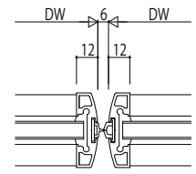
両開き突合せ部
