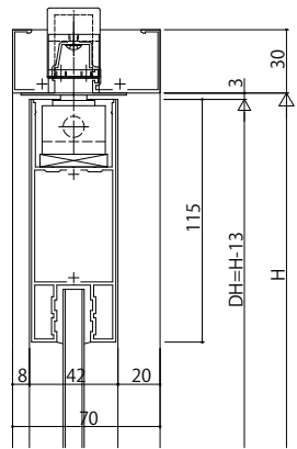
ランマなしの場合
