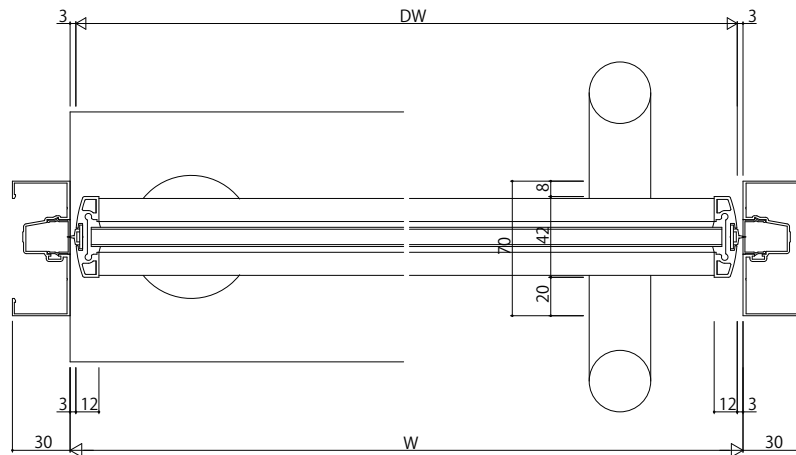
両開き突合せ部
