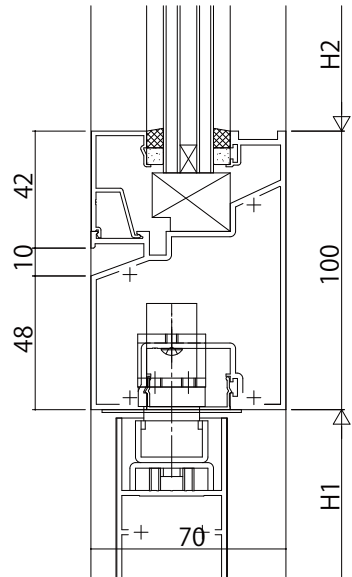
FIX窓/フロアヒンジドア
