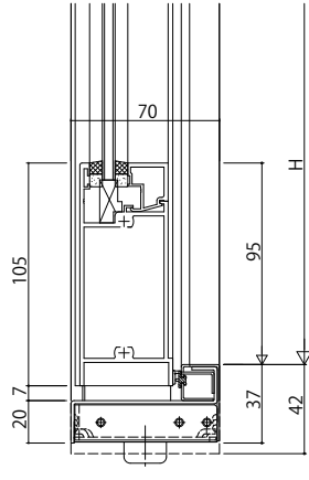
フラット下枠(37見付)
