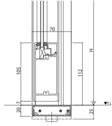
ステンレス下枠(フラット下枠)
