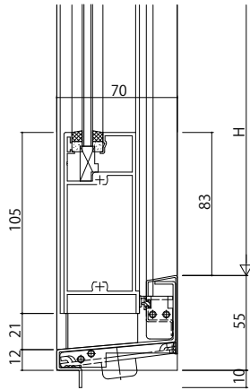
ステンレス下枠
