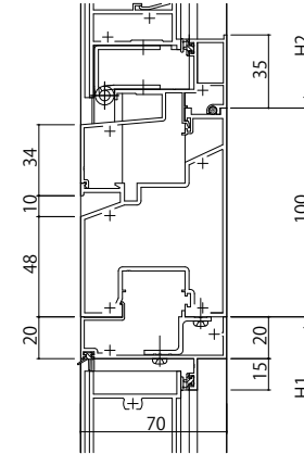
外開し窓/丁番ドア
