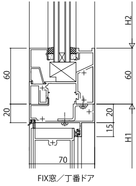
FIX窓/丁番ドア
