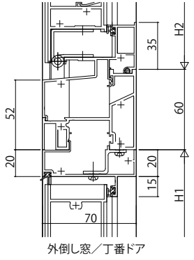
外開し窓/丁番ドア
