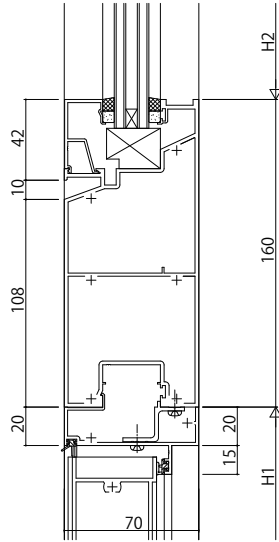
FIX窓/丁番ドア
