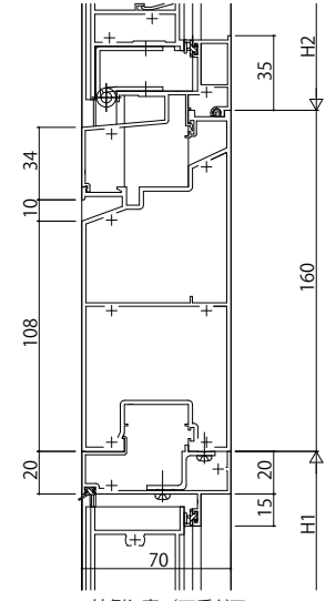
外開し窓/丁番ドア
