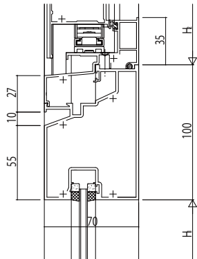
たてすべり出し窓/FIX窓
