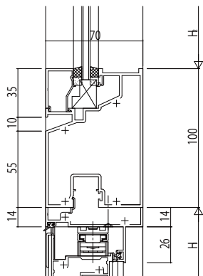
たてすべり出し窓/FIX窓
