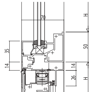
たてすべり出し窓/FIX窓
