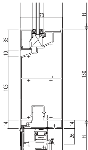
たてすべり出し窓/FIX窓
