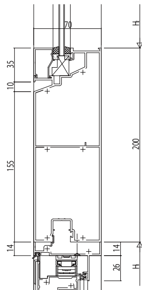
たてすべり出し窓/FIX窓
