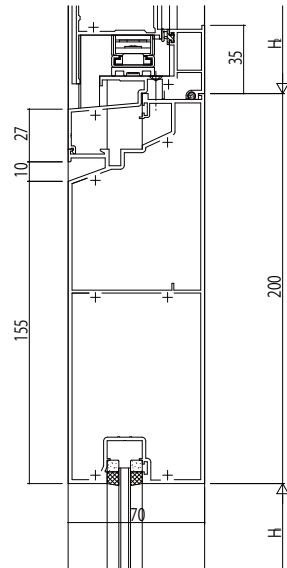
たてすべり出し窓/FIX窓
