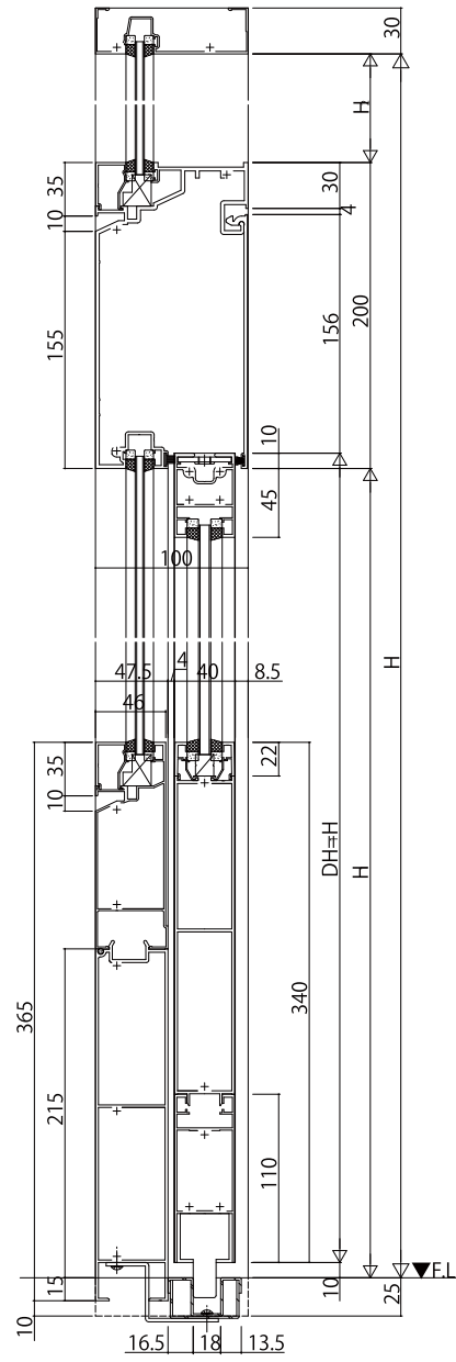
FIX窓/自動ドア 幅木高さ135mm
