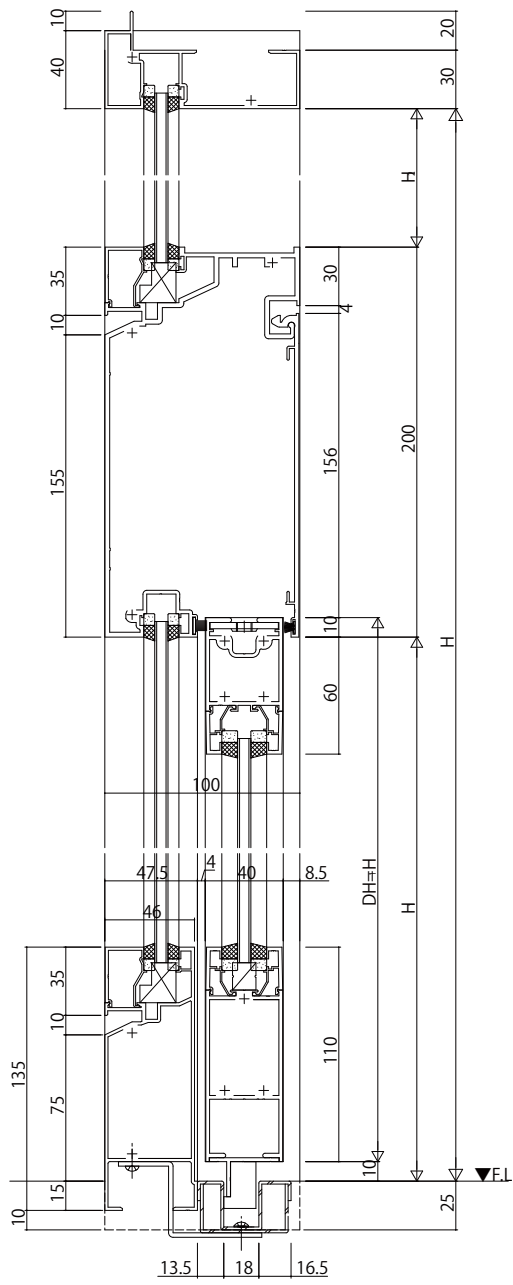
135mm見付幅木 FIX窓/自動ドア
