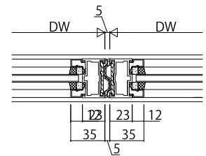
引分け突合せ部
