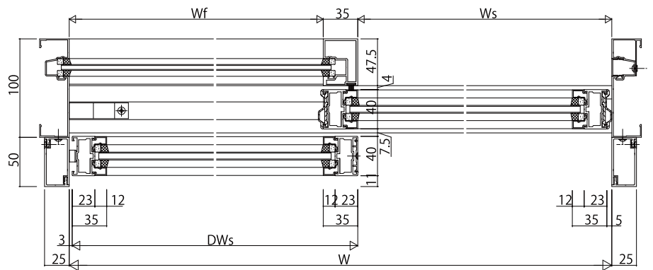
防護スクリーン付自動ドア
