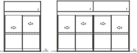
◇割方立35見付・戸先框35見付・縦骨35見付
