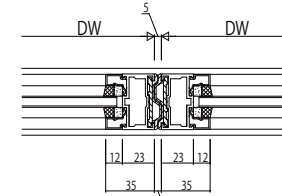
引分け突合せ部
