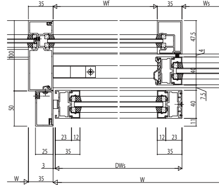
◇割方立35見付・戸先框35見付・縦骨35見付
