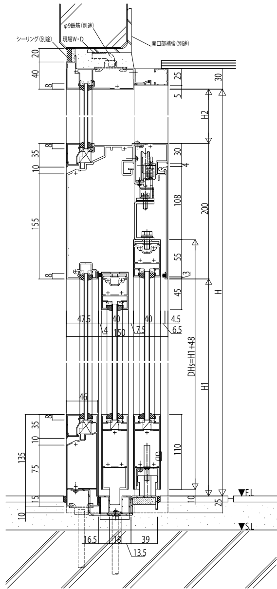
FIX窓/防護スクリーン付自動ドア【一般スライド】
