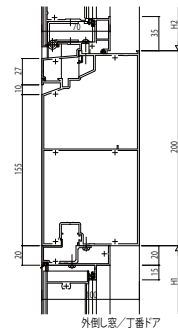
外開し窓/丁番ドア
