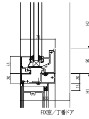
FIX窓/丁番ドア
