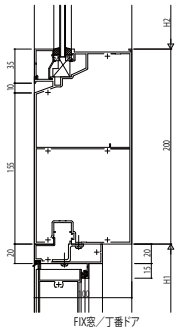
FIX窓/丁番ドア
