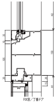
FIX窓/丁番ドア
