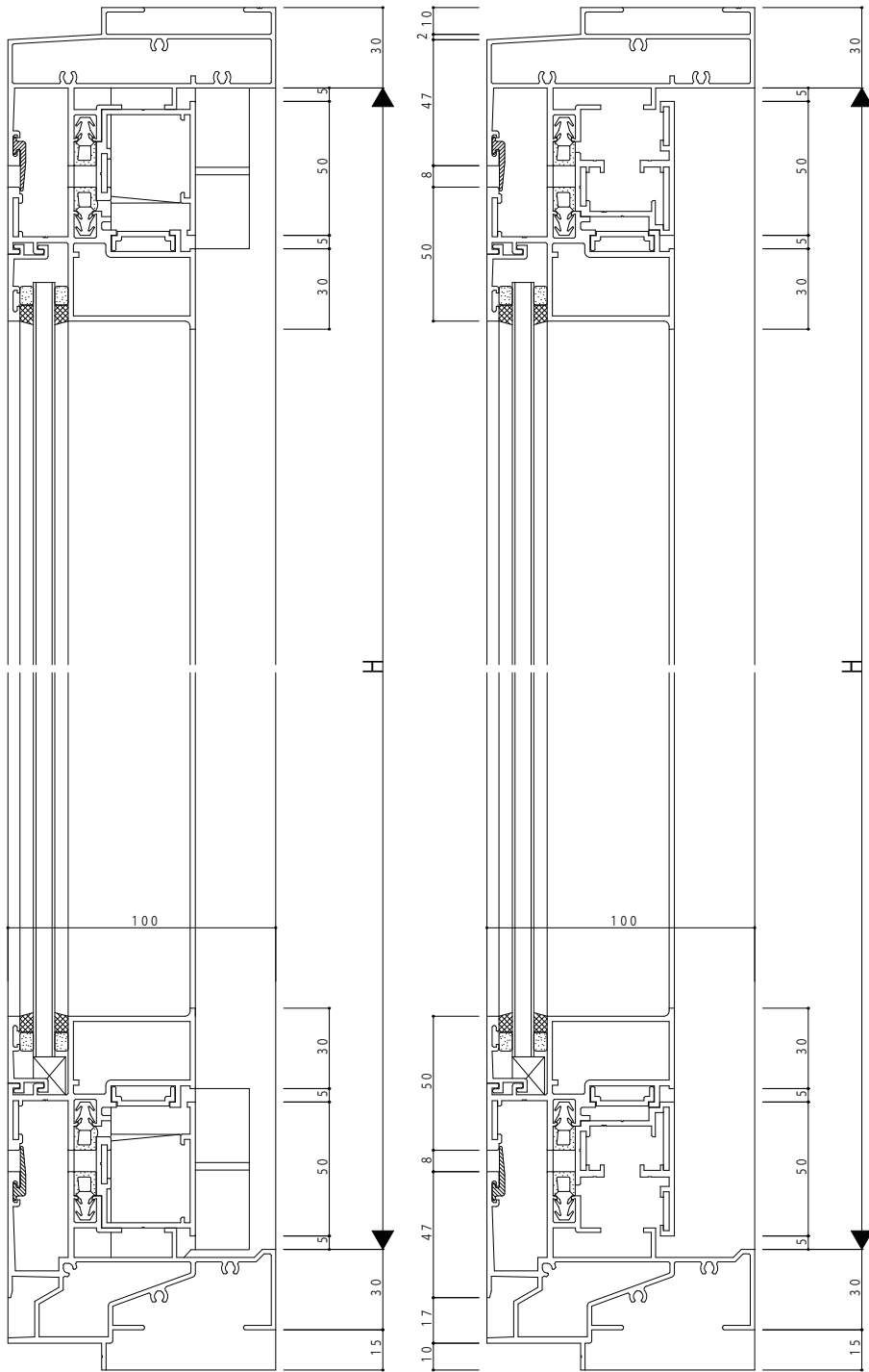
内観:外開き側の断面図
