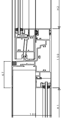
(3) 片引き / F I X 自由片引き / F I X
